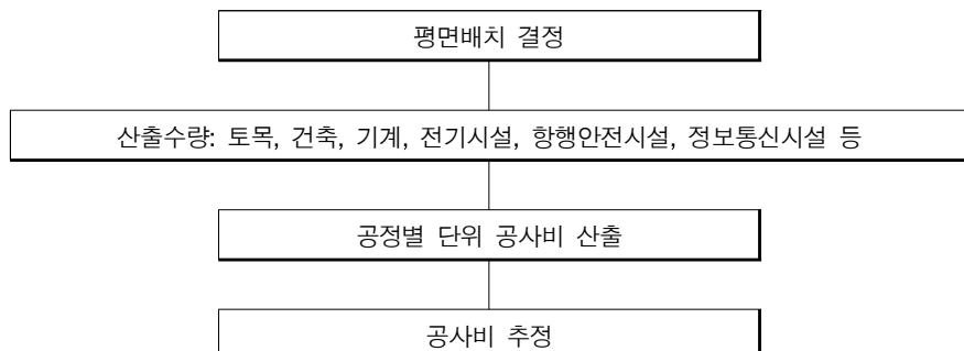
그림 5-5 ■ 공항부문의 공사비 산정 흐름도
