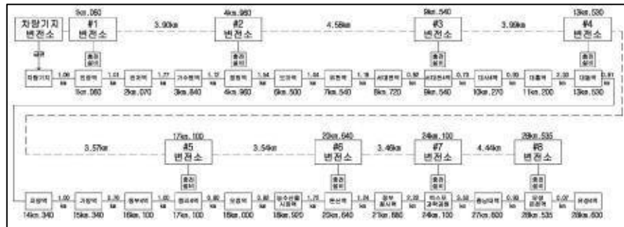
그림 | 급전계통도
