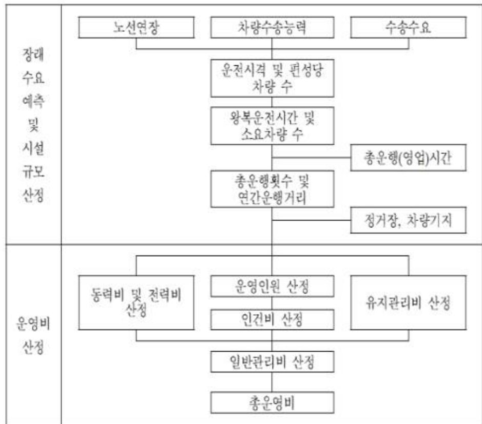
그림 5-6 ■ 노면전차 운영비 추정절차
